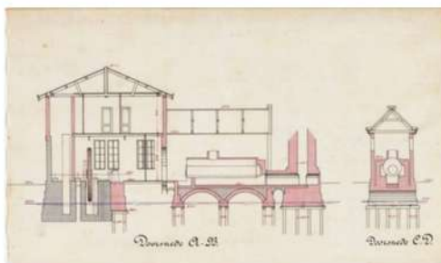
Ontwerptekening Putter Stoomgemaal met de machinistenwoning boven de machinekamer in de onderbouw van het af te breken windgemaal. Dit ontwerp is niet uitgevoerd.
